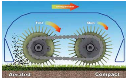
PRINCIPE AERATOR GKB
